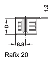
Rafix 20
